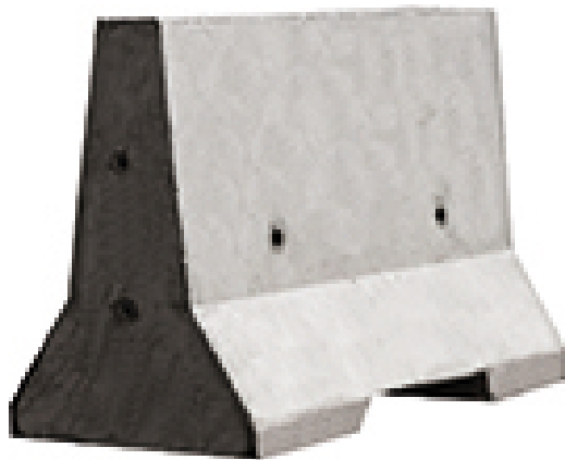
نیوجرسی، معمولی نوع اتصال: با میلگرد ارتفاع 120CM طول 200CM عرض پاشنه 500CM عرض پایه 200CM
